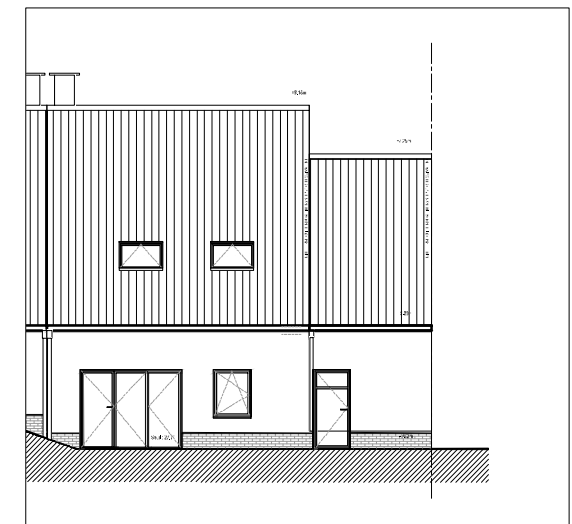
Façade Arrière Ech:1/200 ème
