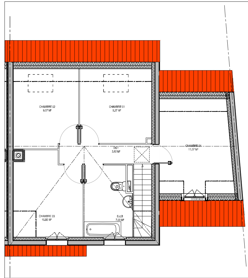
Plan de l'Etage Ech:1/100 ème
