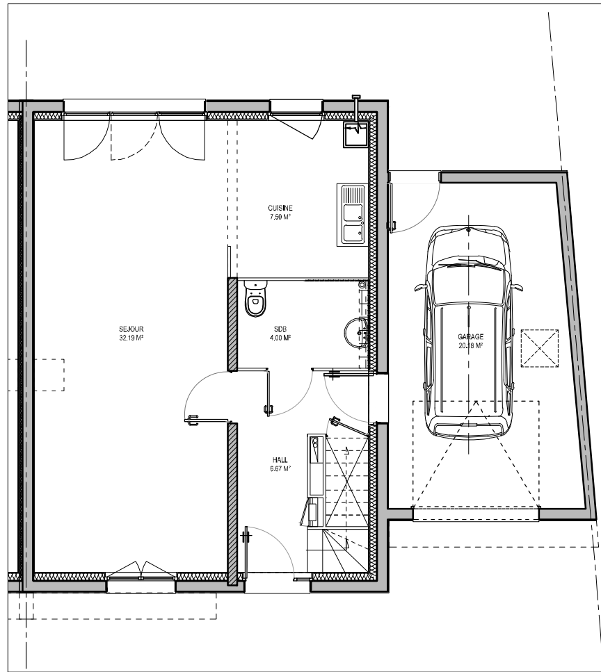
Plan du Rez-de-Chaussée Ech:1/100 ème
