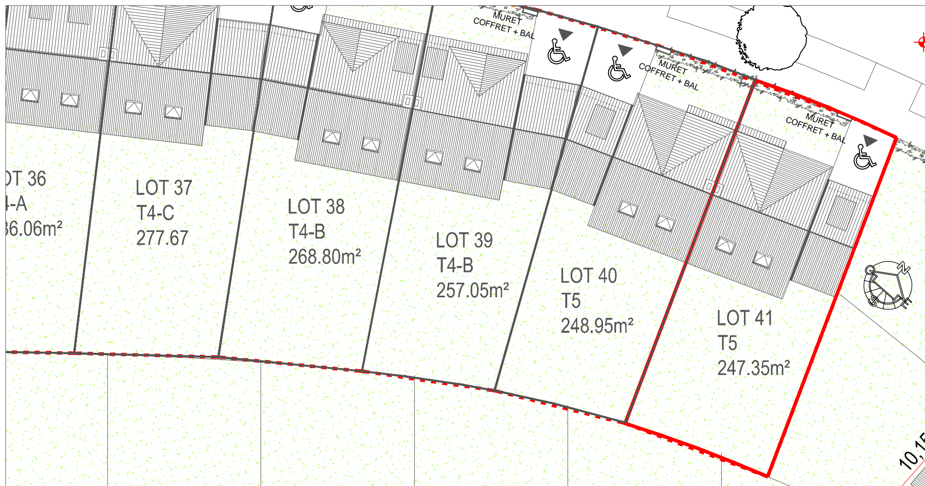
Plan Masse
